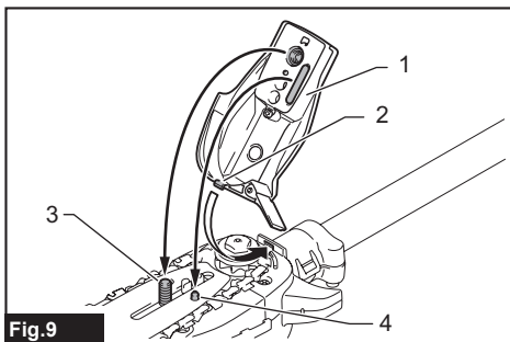
Fig. 9 ► 1. Protecteur de pignon 2. Partie saillante 3. Boulon 4. Broche
