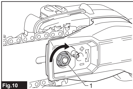
Fig. 10 ► 1. Écrou de retenue
