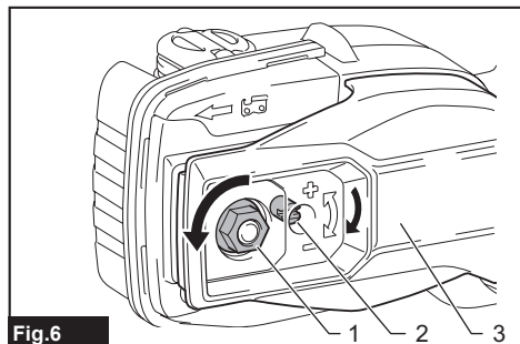
Fig. 6 ► 1. Écrou de retenue 2. Vis de réglage de la chaîne 3. Protecteur de pignon
